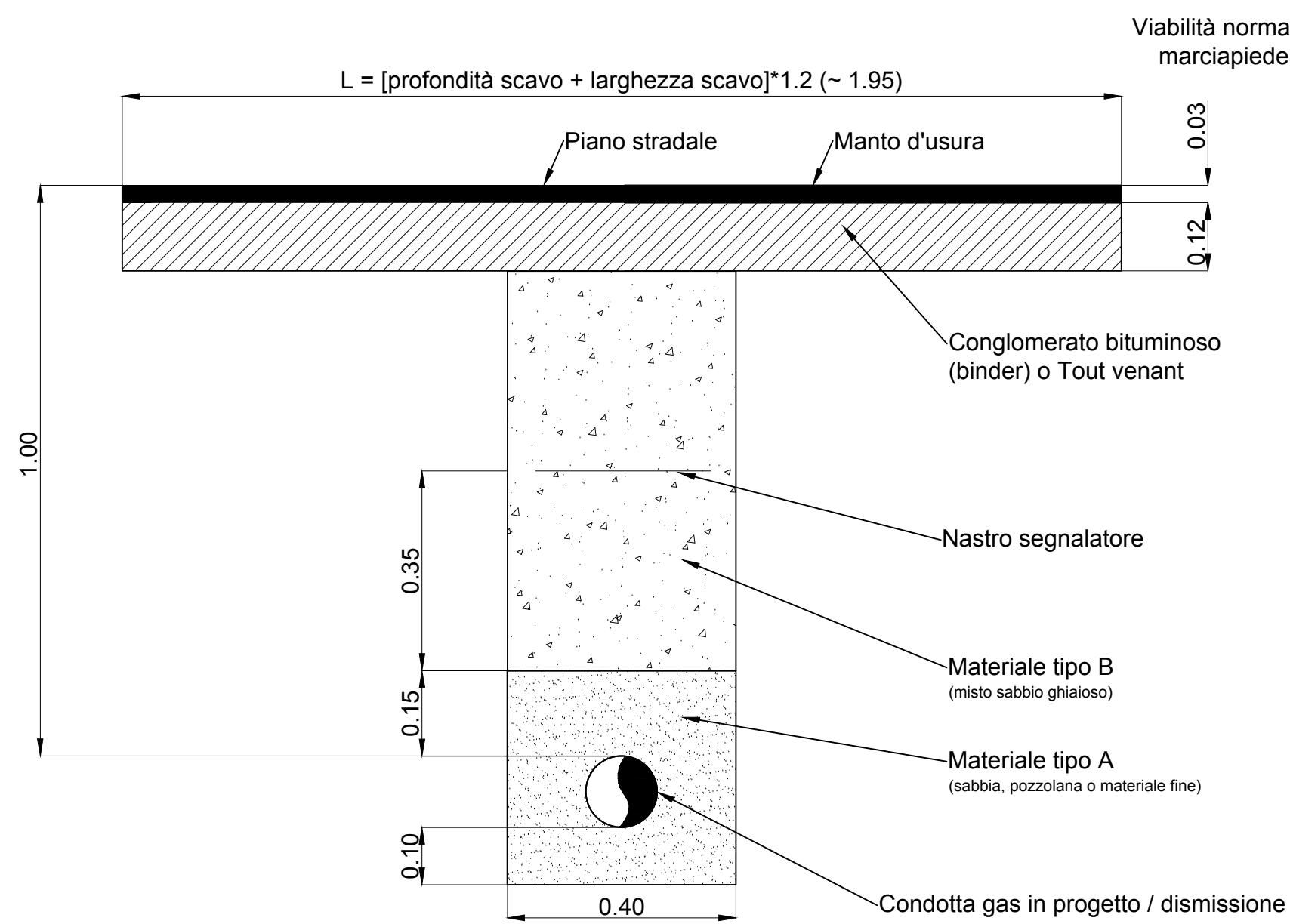
Sezione tipo percorrenza/attraversamento marciapiede strada comunale asfaltata Condotta gas in progetto/dismissione Pe De 125/ GH DN 100
