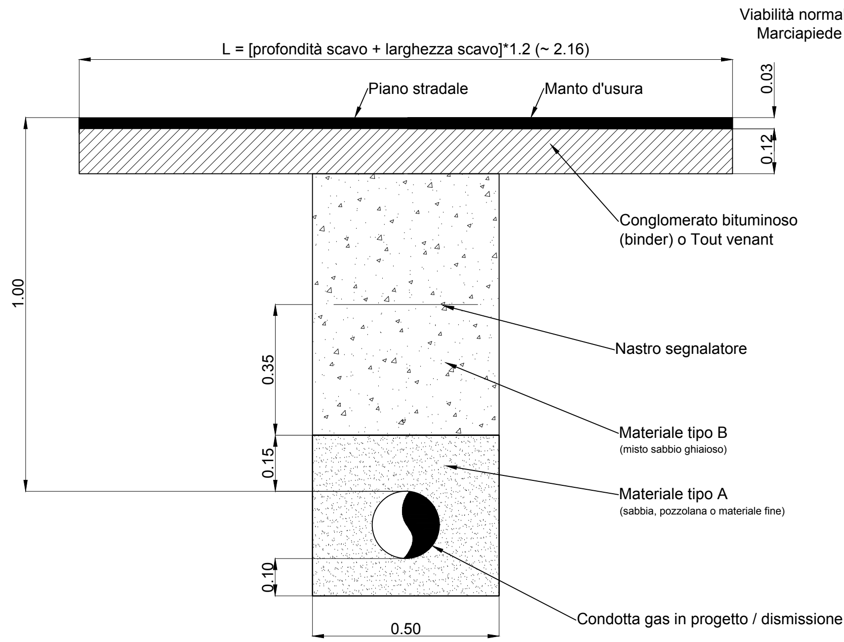
Sezione tipo percorrenza/attraversamento marciapiede strada comunale asfaltata Condotta gas in progetto/dismissione Pe De 180/ ACC-GH DN 150/GH DN 200/Pe De 225/ ACC DN 200
