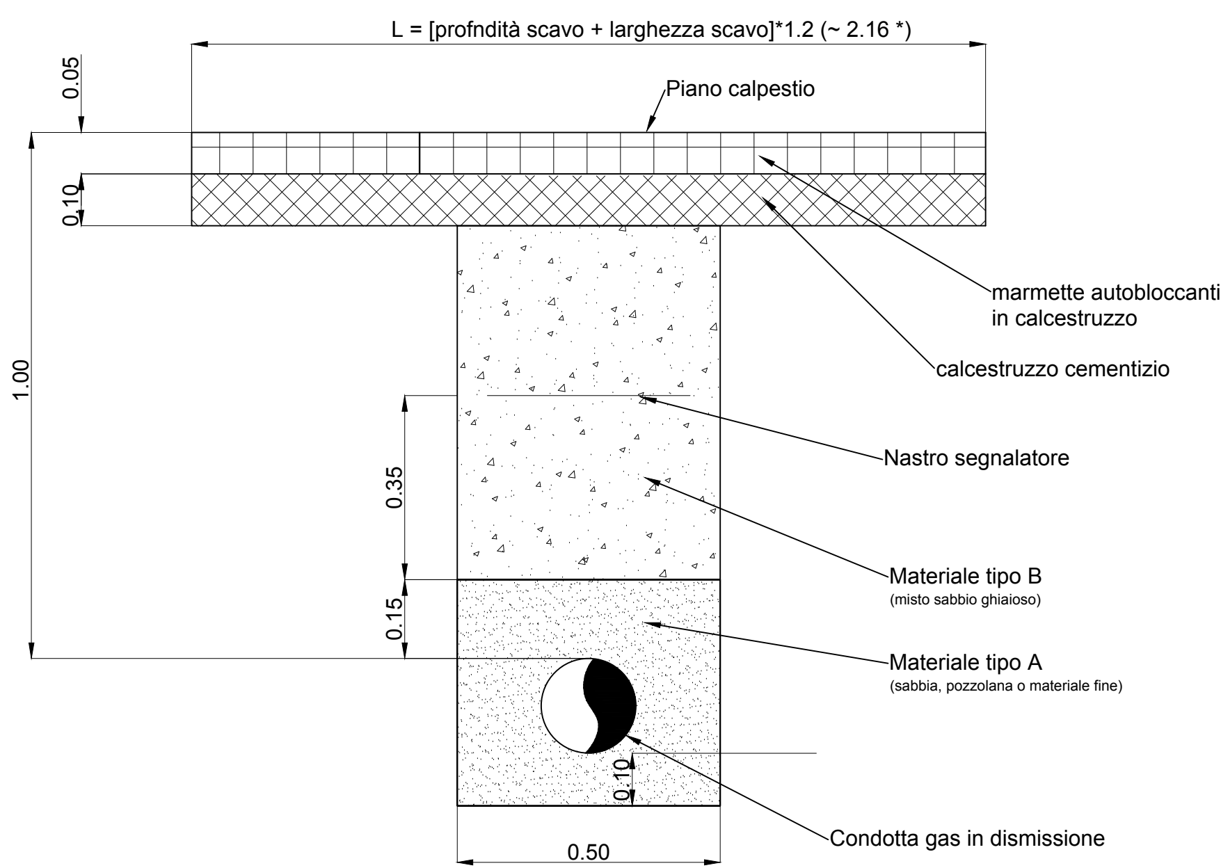
Sezione tipo pavimentazione autobloccanti Condotta gas in dismissione Pe De 180
