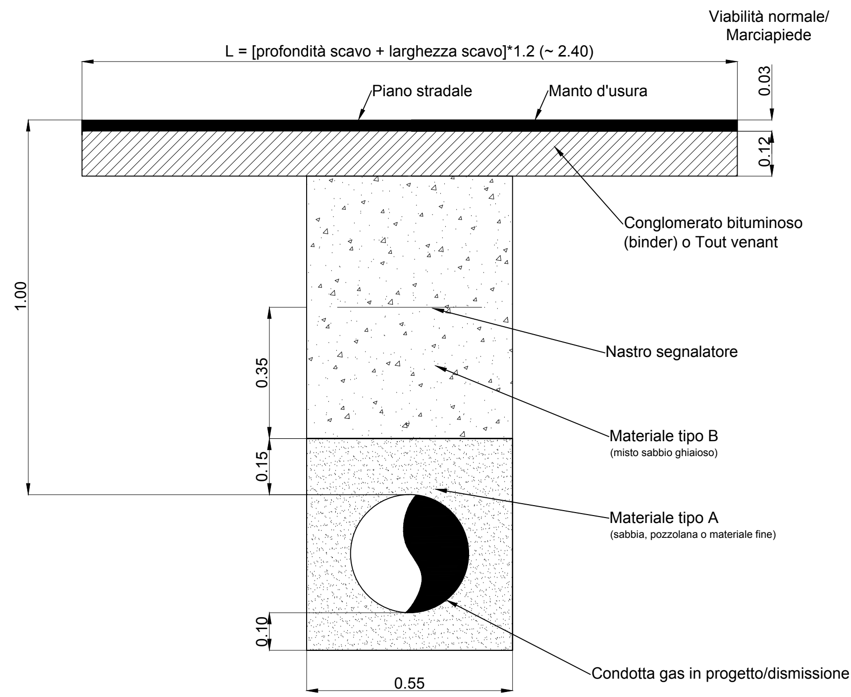
Sezione tipo percorrenza/attraversamento marciapiede strada comunale asfaltata Condotta gas in progetto/dismissioni Pe De 315/ GH DN 300/GH DN 250
